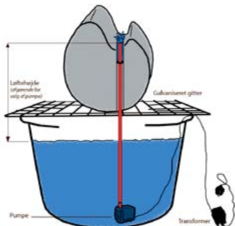
Installation af pumpe uden lys i bassin/balje med galvaniseret gitter.
